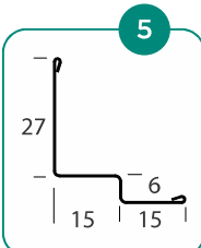
sectiune W 27 x 15 x 6 x 15 mm
