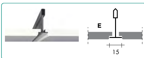
muchie E15 - structura retrasa
